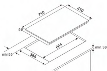
感應爐安裝圖
